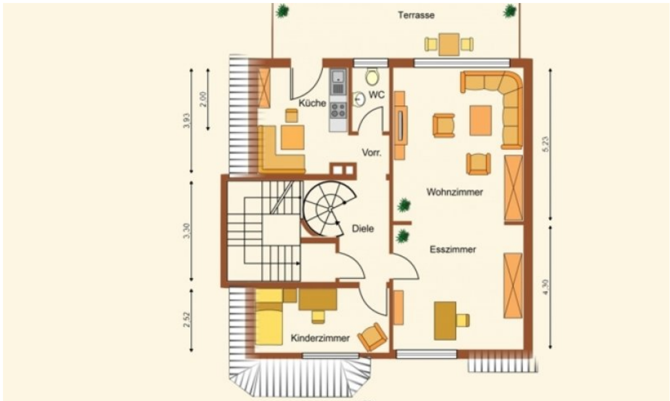
Obergeschoß (Grundriss)
